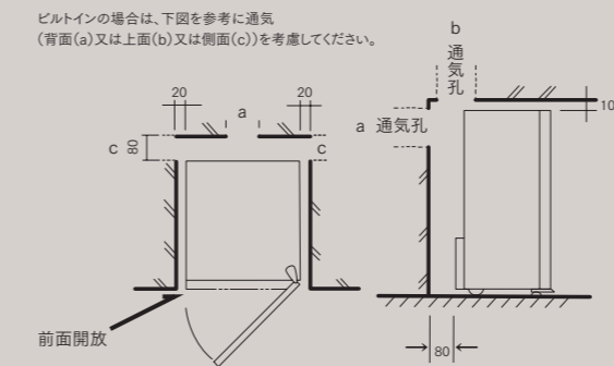
[図1-1] レヴェラシオン、ピュア、プルミエシリーズ、コンパクト59（259サイズ）、6000
